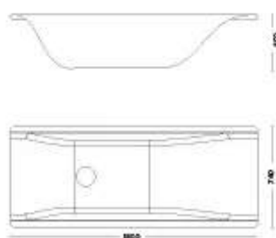
VASCA DA INCASSO INSET BATH TUB 1800x740
