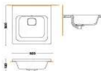
LAVABO 50 WASHBASIN 50 SONE.10.01
