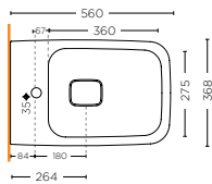
BIDET FILO MURO BACK TO WALL BIDET SCLB.30.F01
