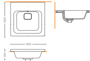
LAVABO 50 WASHBASIN 50 SONE.10.01
