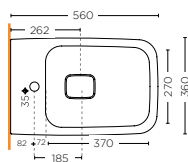
BIDET SOSPESO WALL HUNG BIDET SCLB.30.W01
