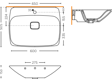
LAVABO 65 CM WASHBASIN 65 CM SCLB.10.01
